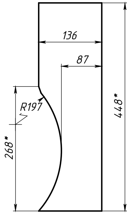
Поз.2 (Угольник) развертка
