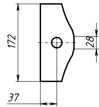
Поз.4 (Ушко) развертка
