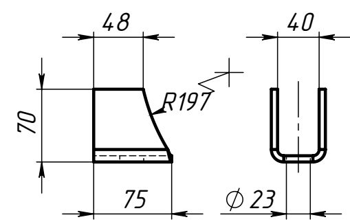
Поз.4 (Ушко)
