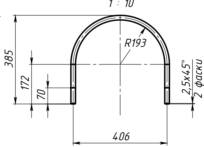
Поз.5 (Хомут) 1 : 10
